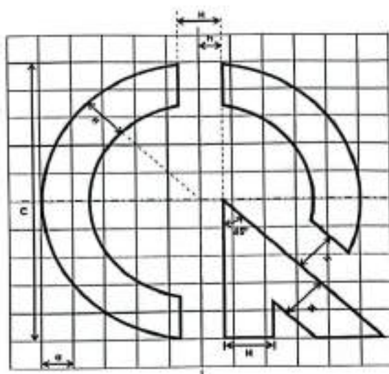
Hình 02. Kích thước cơ bản của dấu hợp quy
